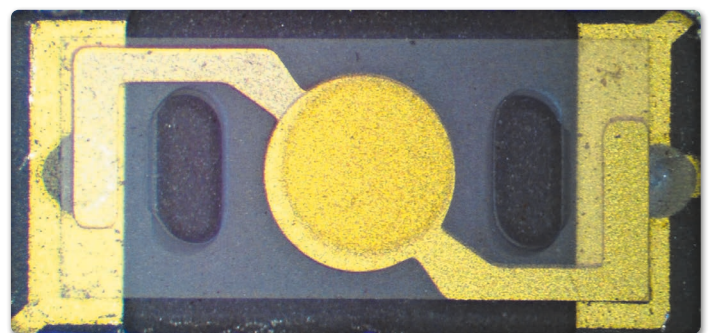
Bild 1: Die Struktur des Bi-MESA-Podestes
