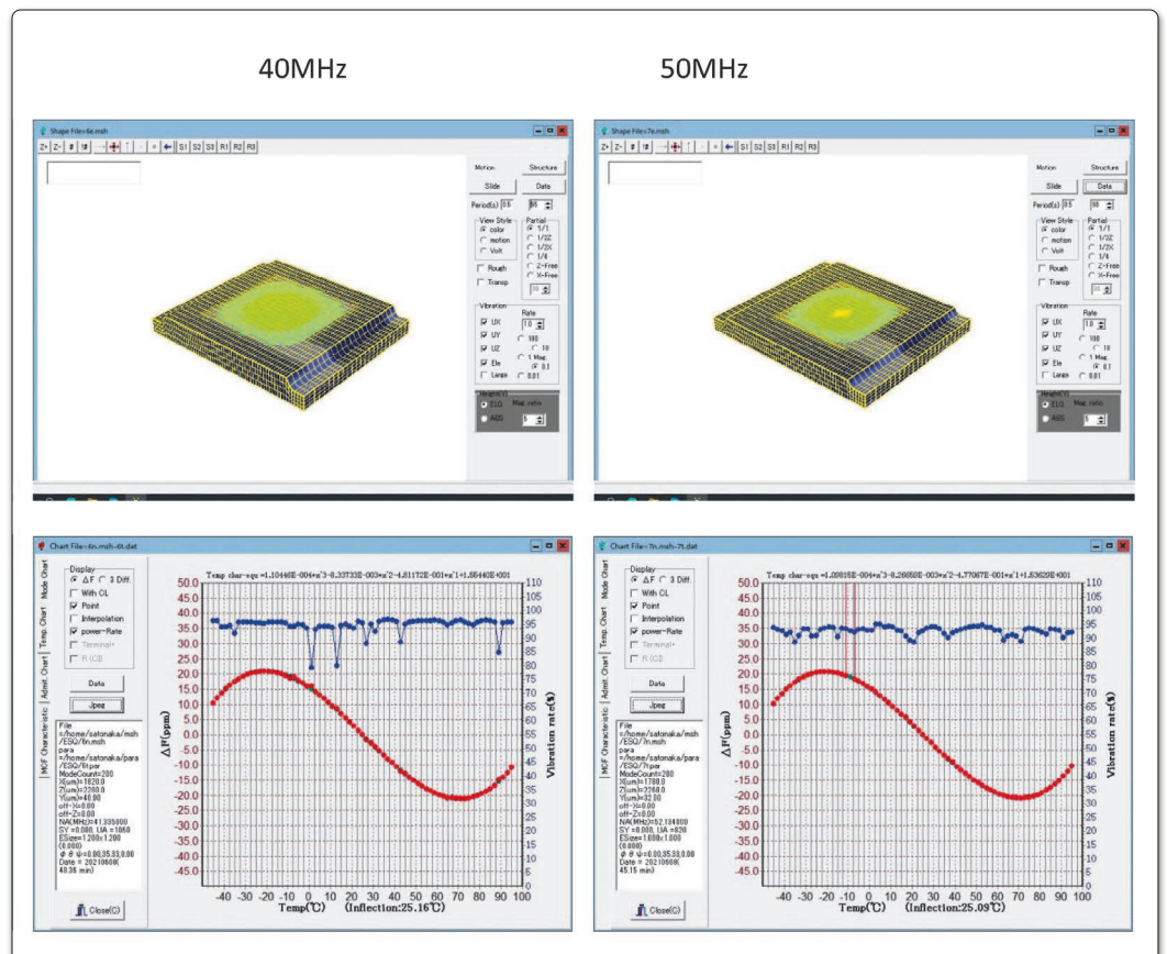
Bild 4: Die Dimensionen des Quarz-Blanks wurden simuliert und optimiert
