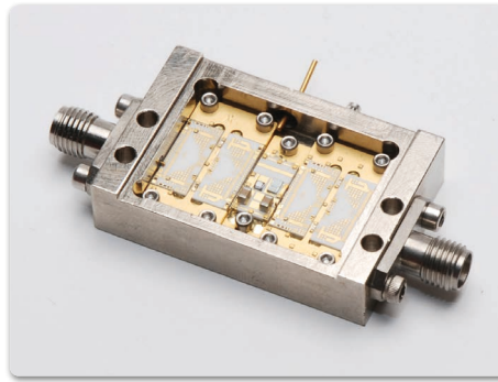
Benchtop-Verstärker
