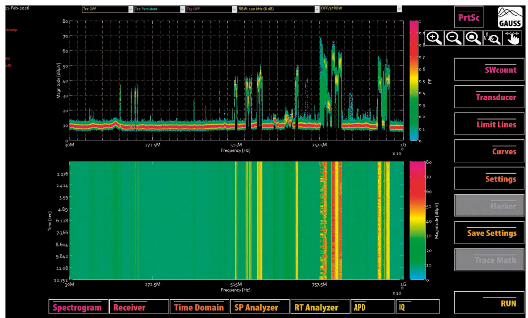
Bild 5: Ultra-high resolution Persistence Mode mit 1 GHz Bandbreite
