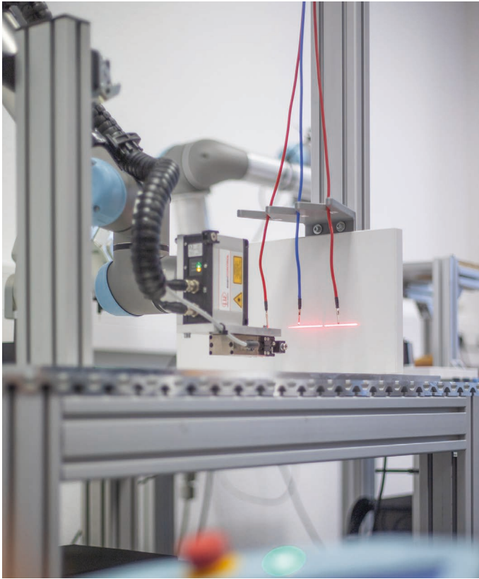
Bild 2: Roboter in Kombination mit Sensoren und moderner Programmiersoftware eröffnen ganz neue Automatisierungsmöglichkeiten. © ArtiMinds Robotics GmbH
