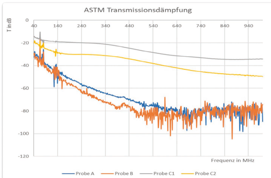
Bild 2: EMV-Messungen nach ASTM ES 7/83 verschiedener Carbonfaser/PA6-Proben
