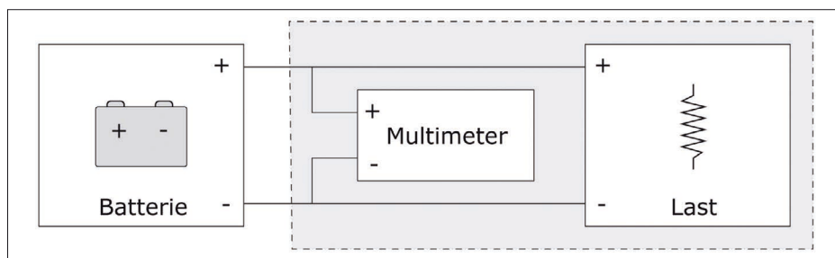
Bild 2: Aufbau zum Entladen einer Batterie mit einer elektronischen Last
