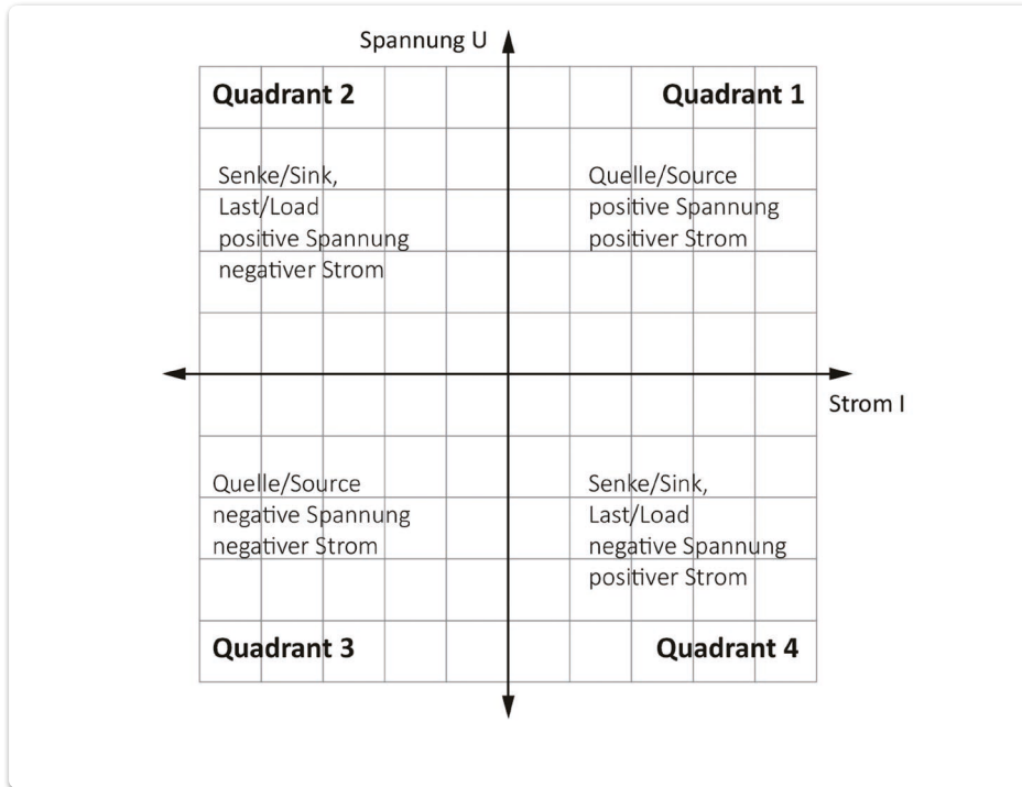
Bild 1: Das 4-Quadrant-Modell für Stromquellen und -senken
