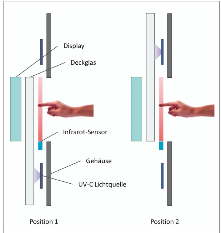
Bild 3: Hygienischer Touchscreen mit automatischer Desinfektion (© HY-LINE Computer Components )
