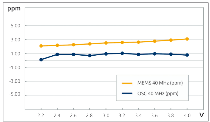
Bild 7: Vergleich der Start-Up-Charakteristik von MEMS- und Quarz-Oszillatoren bei 40 MHz
