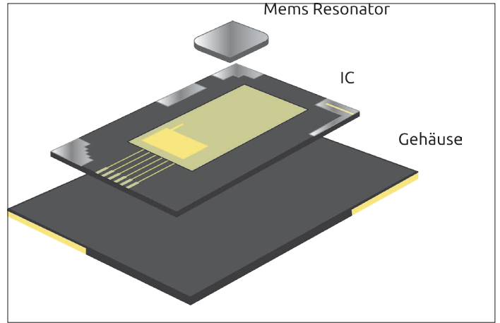
Bild 4: Typischer Aufbau eines MEMS-basierten Oszillators
