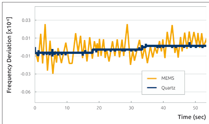
Bild 9: Vergleich der Frequenzstabilität von Quarz- und MEMS-Oszillator
