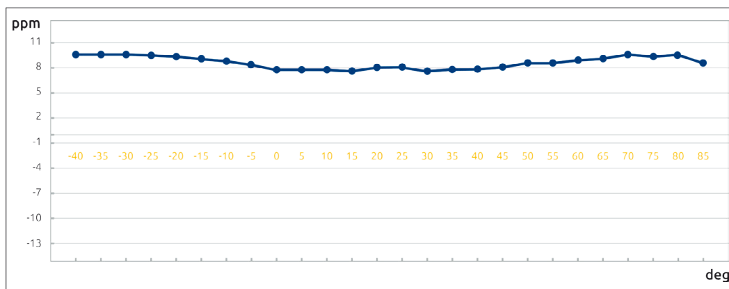
Bild 10. Frequenzstabilität über den Arbeitstemperaturbereich bei 40 MHz, a) Quarzoszillator, b) MEMS-Oszillator
