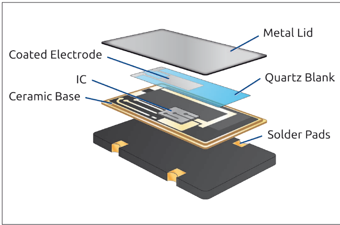
Bild 3: Typischer Aufbau eines quarzbasierten Oszillators
