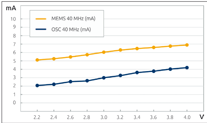
Bild 6: Vergleich der Stromaufnahme von MEMS- und Quarz-Oszillatoren bei 40 MHz
