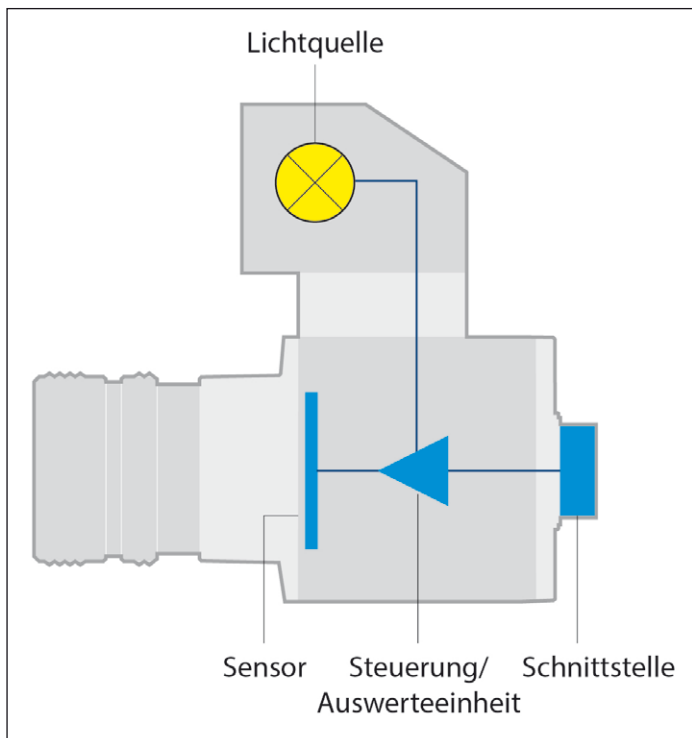
Bild 1: Komponenten der Time-of-Flight-Kamera
