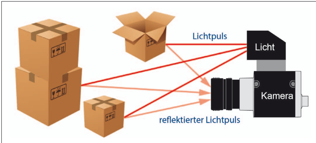
Bild 2: Funktionsprinzip der Lichtlaufzeit-Kamera
